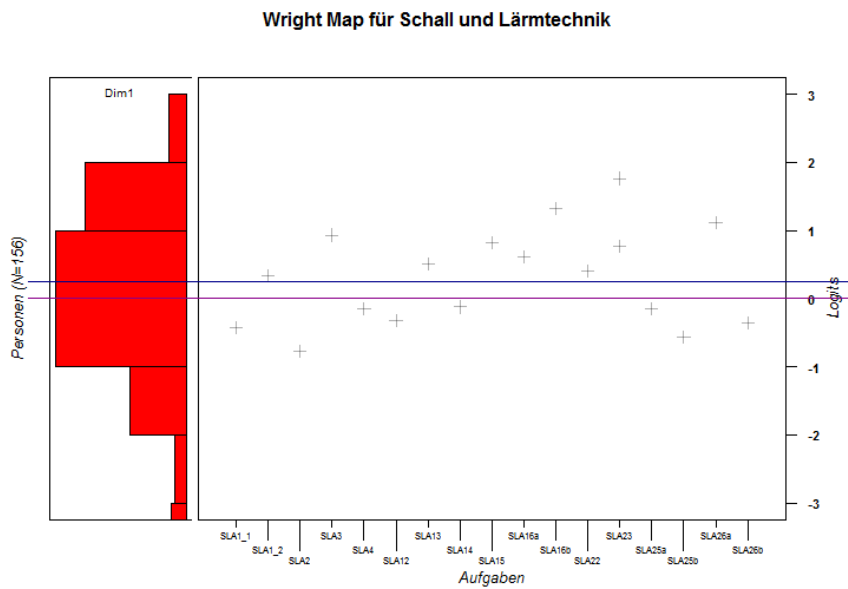
Abbildung 9: Darstellung der Wright Map für den Test Schall und Lärmtechnik
