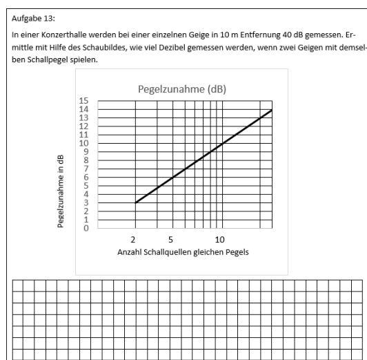
Abbildung 10: Item SLA13 zum Test Schall- und Lärmtechnik
