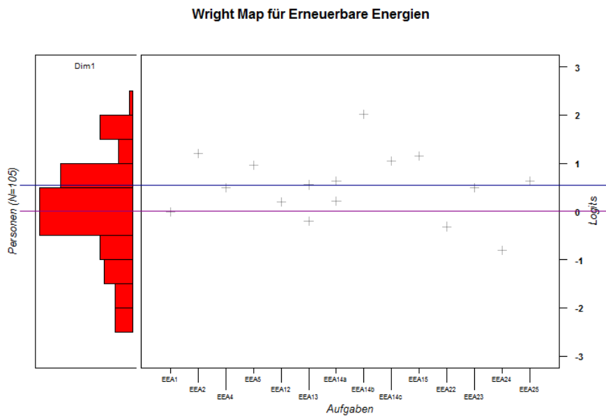
Abbildung 5: Darstellung der Wright Map für den Test Erneuerbare Energien
